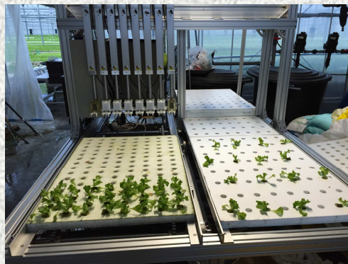
☆野菜移植機 R II-1
