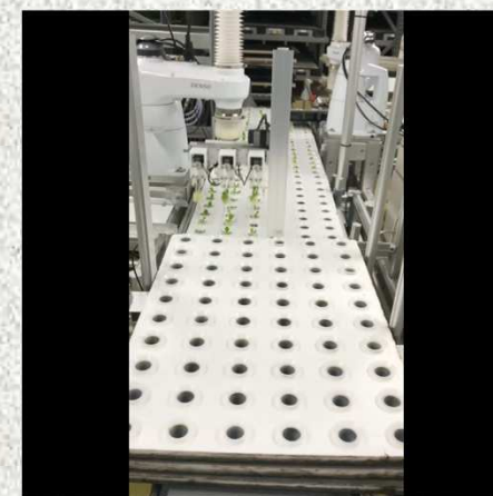
☆野菜移植機 R III 2連タイプ
